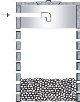
SUMIDOURO (OU POÇO ABSORVENTE)
