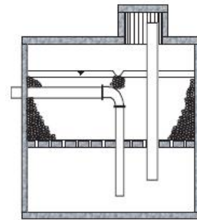
FILTRO ANAERÓBICO (BIOLÓGICO)
